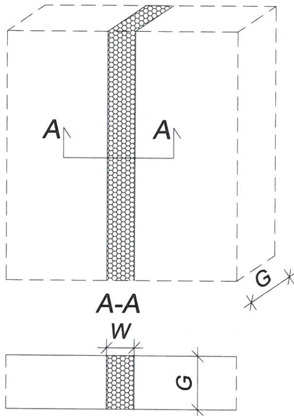
Rys. C1. Widok i przekrój uszczelnia pionowego złącza liniowego w ścianie
