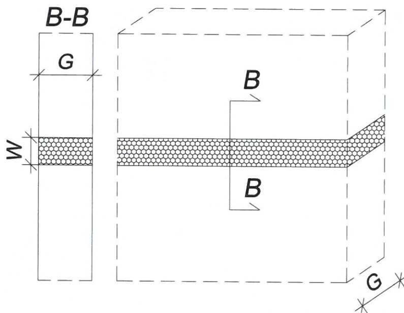
Rys. C2. Widok i przekrój uszczelnia poziomego złącza liniowego w ścianie
